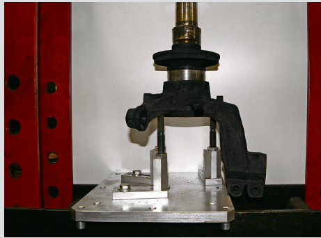
Lager-/Naben-Einheit einpressen
